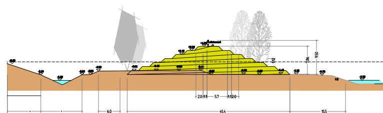
Doorsnede Uitkijkheuvel
