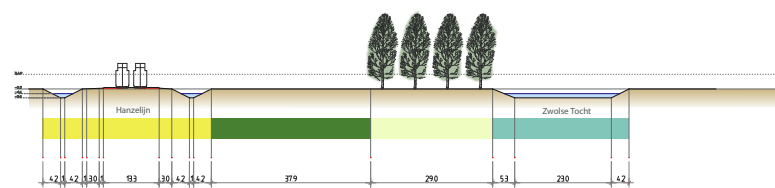
Doorsnede huidige situatie
