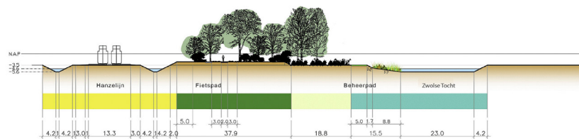
Doorsnede situatie over 10 jaar
